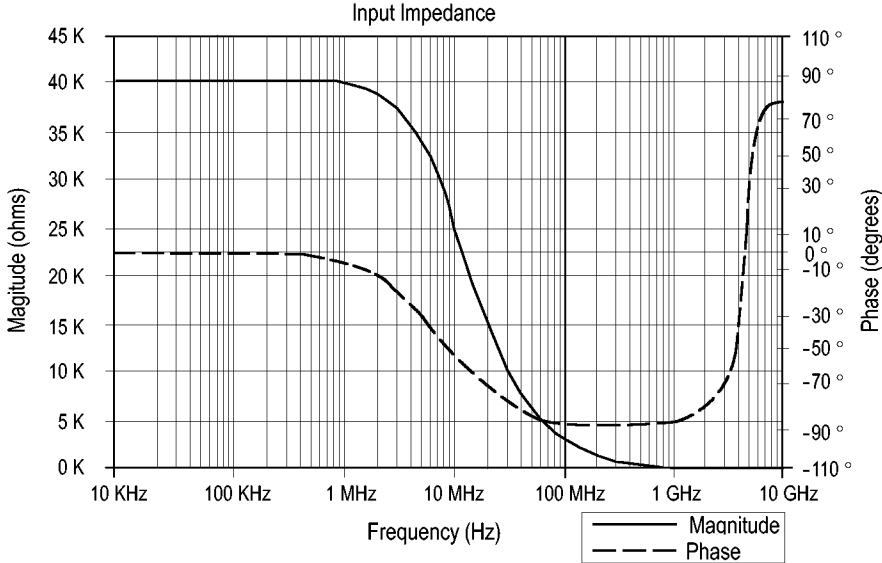
图 4: 典型输入阻抗和相位与频率关系图
